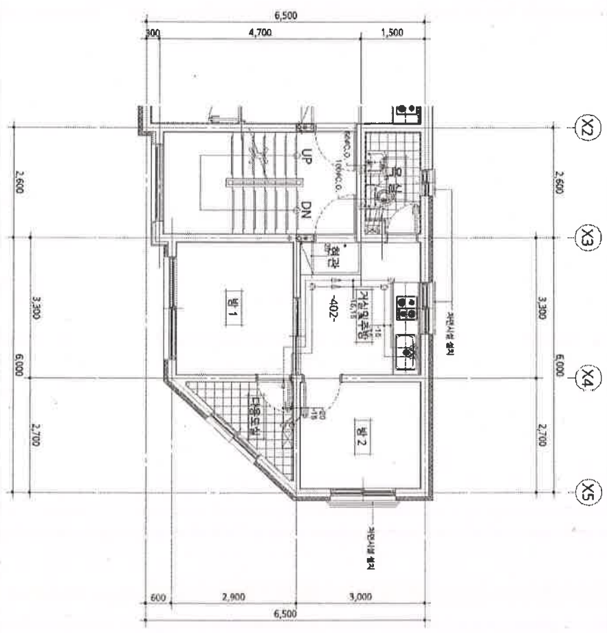
건축물현황도
